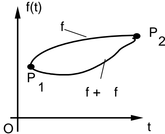
Fig. 2 - Variazioni di isocrone di un funzionale di funzioni dipendenti solo dal tempo
