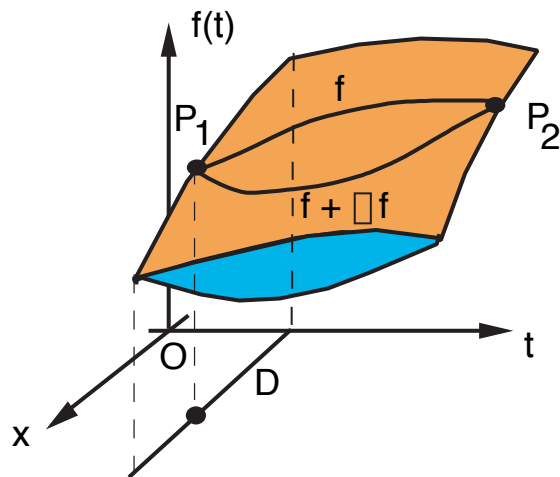
Fig. 3 - Variazioni di isocrone di un funzionale di funzioni dipendenti dal tempo e dalle coordinate
