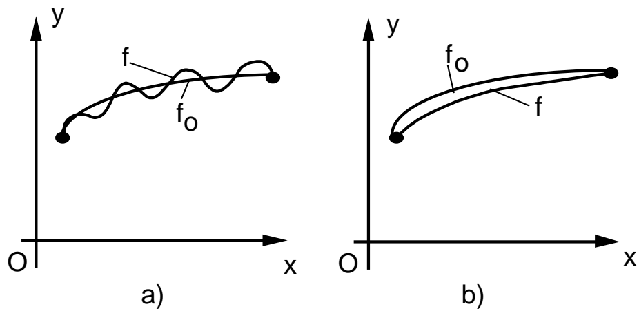
Fig. 1 - Funzionale continuo: a) fino all'ordine 0; b) fino all'ordine n
