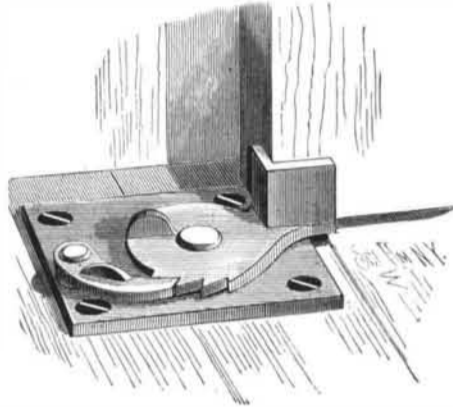
CALLAWAY'S DOOR CHECK OR HOLDER.
