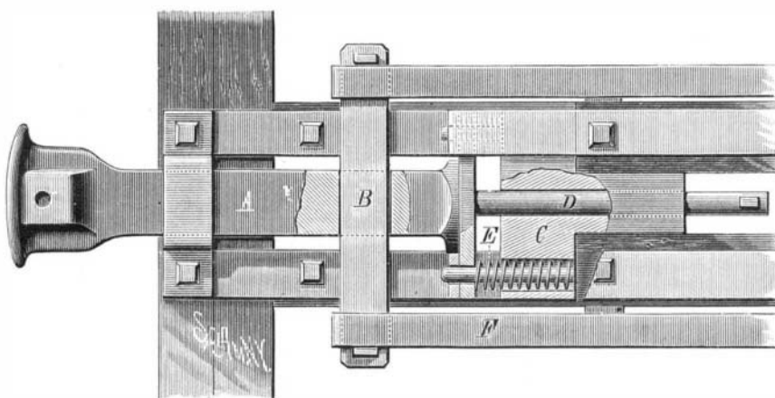
Fig. 3.—DRAW BAR.
