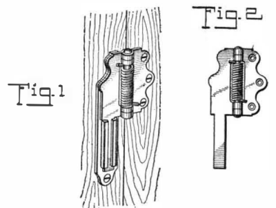
DETACHABLE HINGE.
